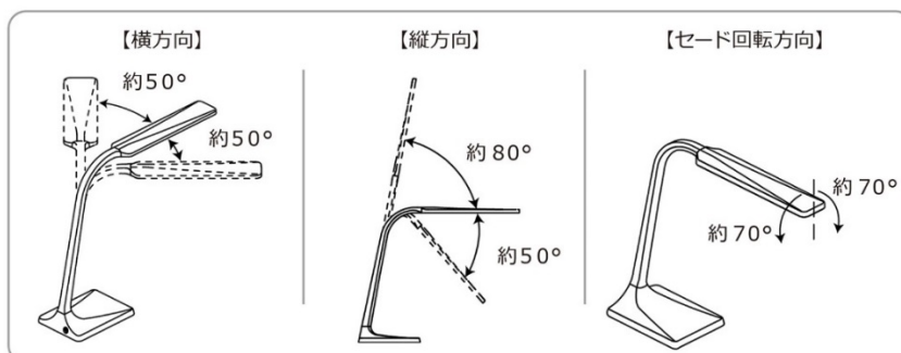
(図3) アームの可動範囲
